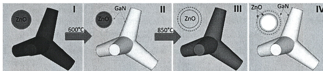
Fig. 5. Ilustrarea schematică a procesului de creștere a aerogalnitului. Etapele ilustrează: (I) un singur microtetrapod de ZnO, (II) creșterea inițială a stratului de GaN la 600 °C, (III) creșterea GaN de înaltă calitate și descompunerea simultană a ZnO la 850 °C și (IV) creșterea de GaN atât pe suprafețele interioare, cât și pe cele exterioare, ducând la formarea unui strat de ZnO îngropat.
