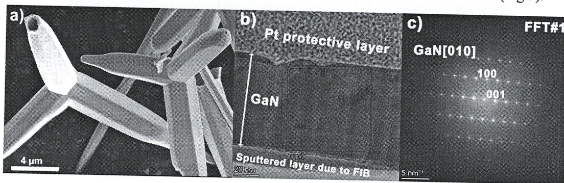
Fig. 3. Imagini SEM a microtuburilor de aero-GaN (a); HRTEM a secțiunii transversale a peretelui microtubului (b) și paternul FFT a regiunii respective (c);
