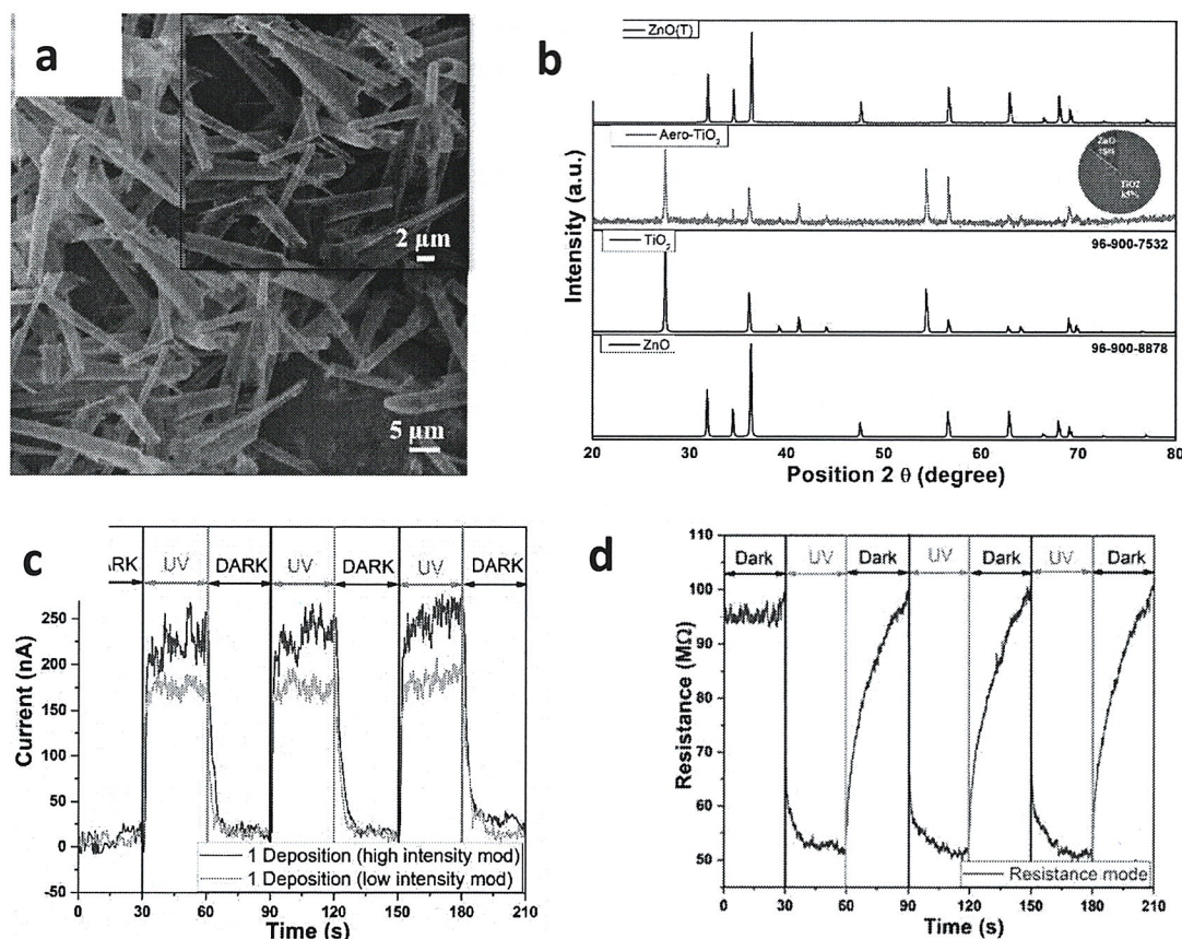
Fig. 1. Imaginea SEM a aero-TiO 2 utilizat în calitate de sensor de UV; (b) Caracteristica XRD a probelor de aero-TiO 2 ; (c), (d) Răspunsul la iluminare cu UV
